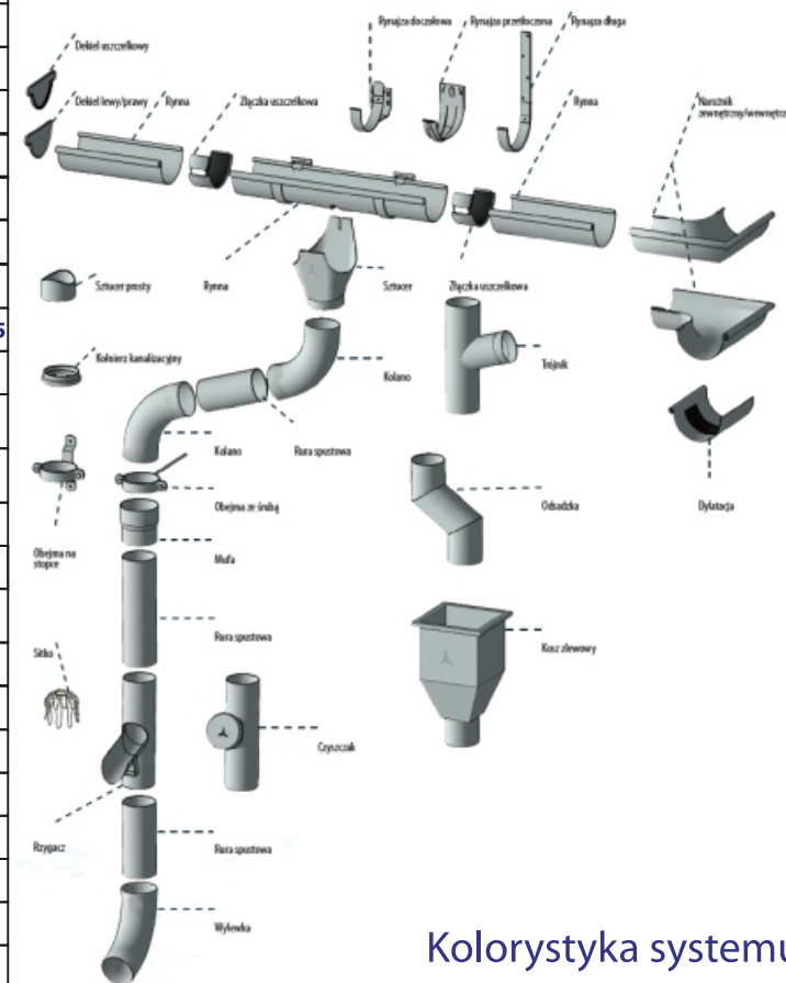
Schemat systemu
